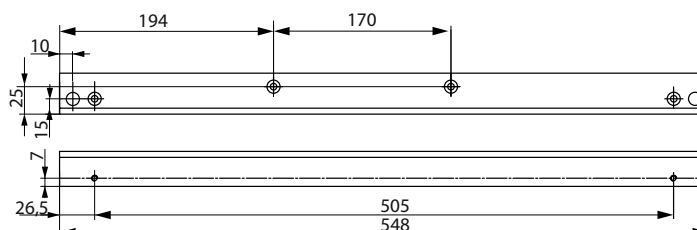
Consolă unghi A116 Pentru brat culisant G460 cu instalare pe partea fără balamale
