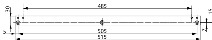
Placă de montaj A115 Pentru brat culisant G460
